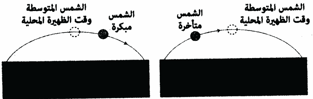
الشكل (89): قمتل الشمس المتوسطة في السماء متوسط زمن الإشعاع الشمسي - أساس ساعاتنا. يمكن للشمس الحقيقية أن تعبر خط الزوال قبل ذلك أو بعده وفق التوقيت في أثناء العام.
